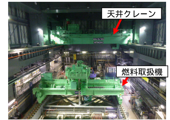
燃料取り出し用カバー内部
