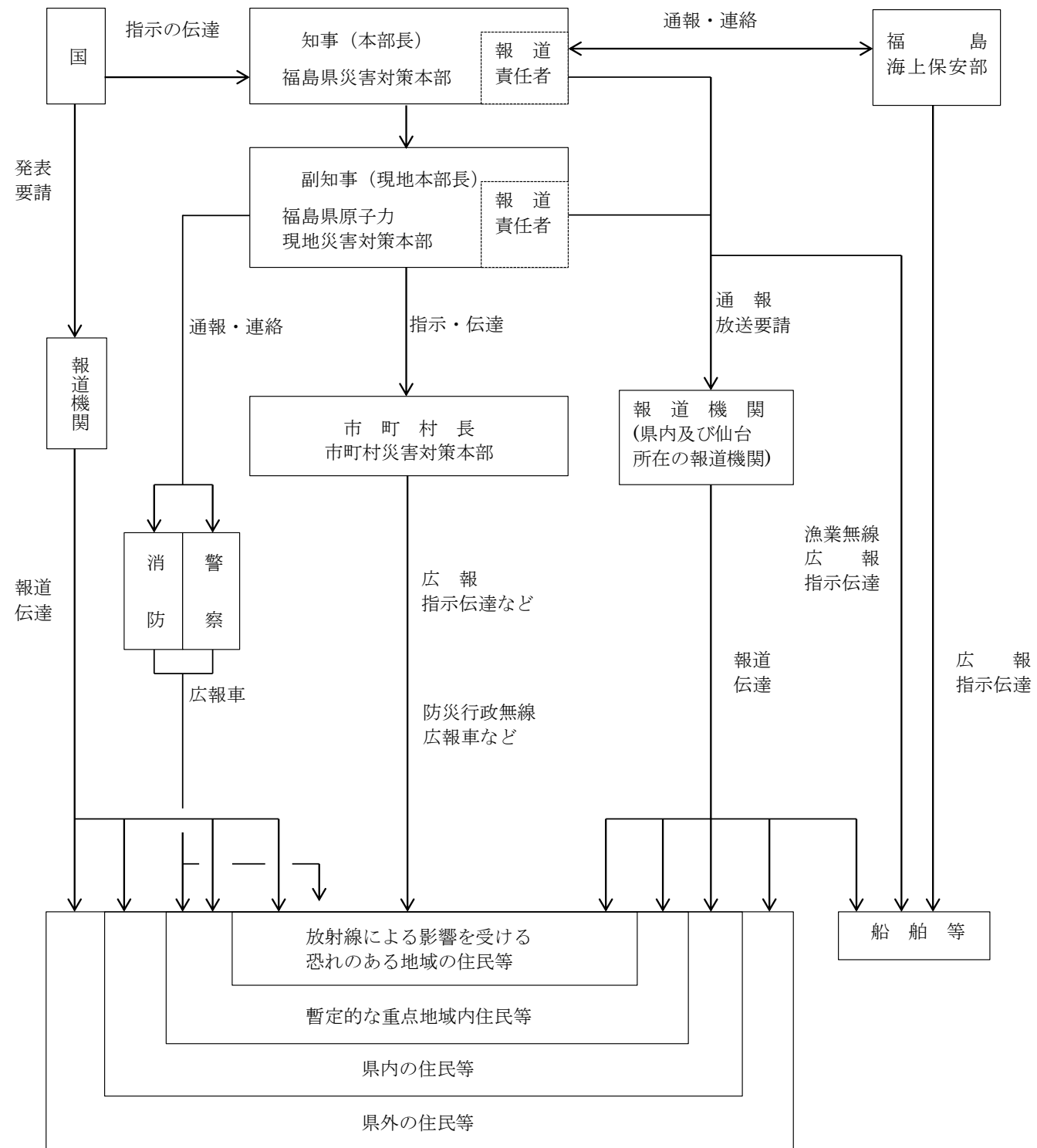
(5) 住民等に対する広報及び指示伝達系統図
