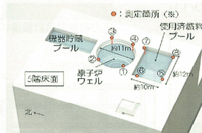
傾きの確認 (水位測定)
