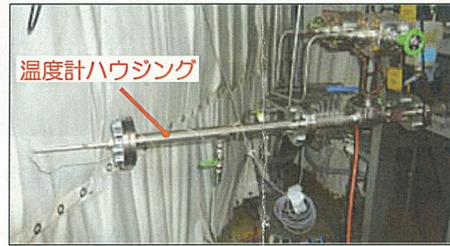
圧力容器温度計設置状況(H24/10/3)
