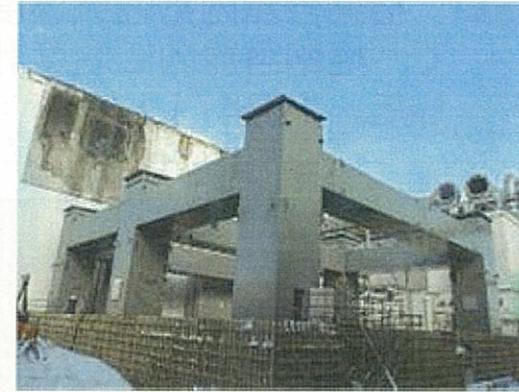
第1節部分鉄骨建方終了 (1/14)
