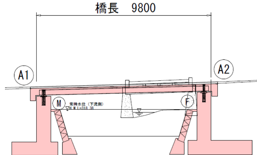
【新町橋側面図】
