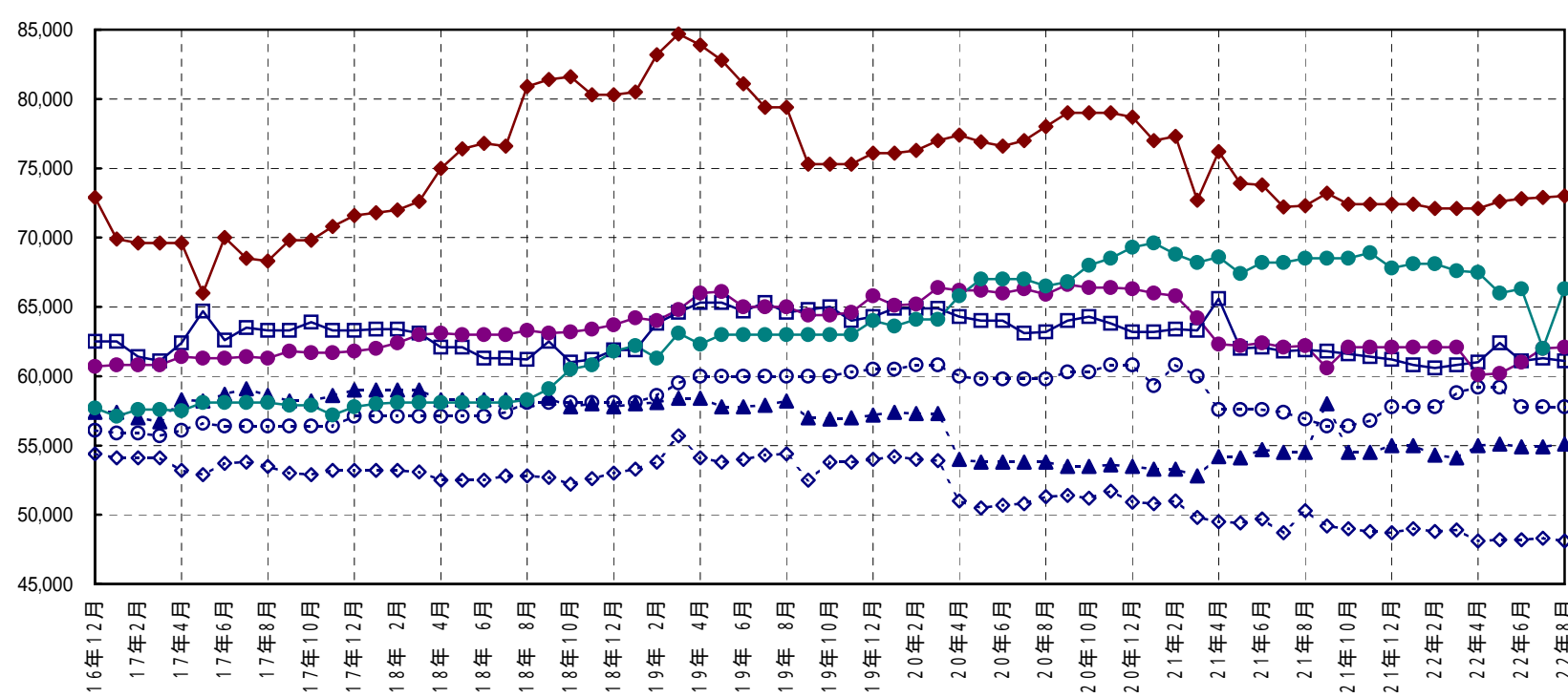
---◇--- スギ正角 □--- スギ正角KD ▲--- アカマツ平角 ○--- 米松正角 ●--- 米松平角 ◆--- 米松平角KD ●--- エゾマツ平角
