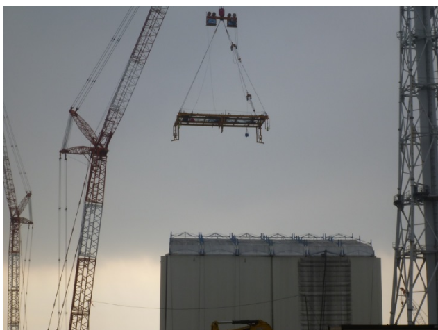
吊上治具を屋根パネル上部に移動している様子
