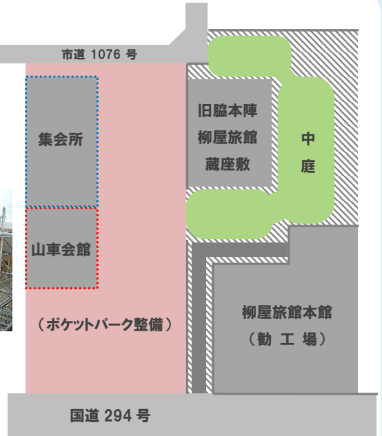
【ポケットパーク配置図】
