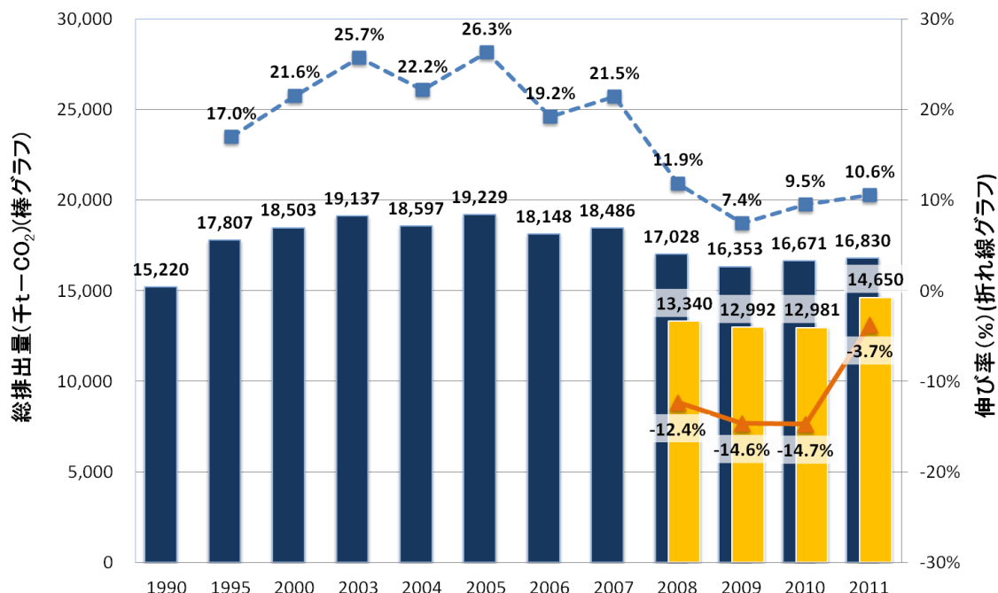
図1 温室効果ガスの排出量及び伸び率
