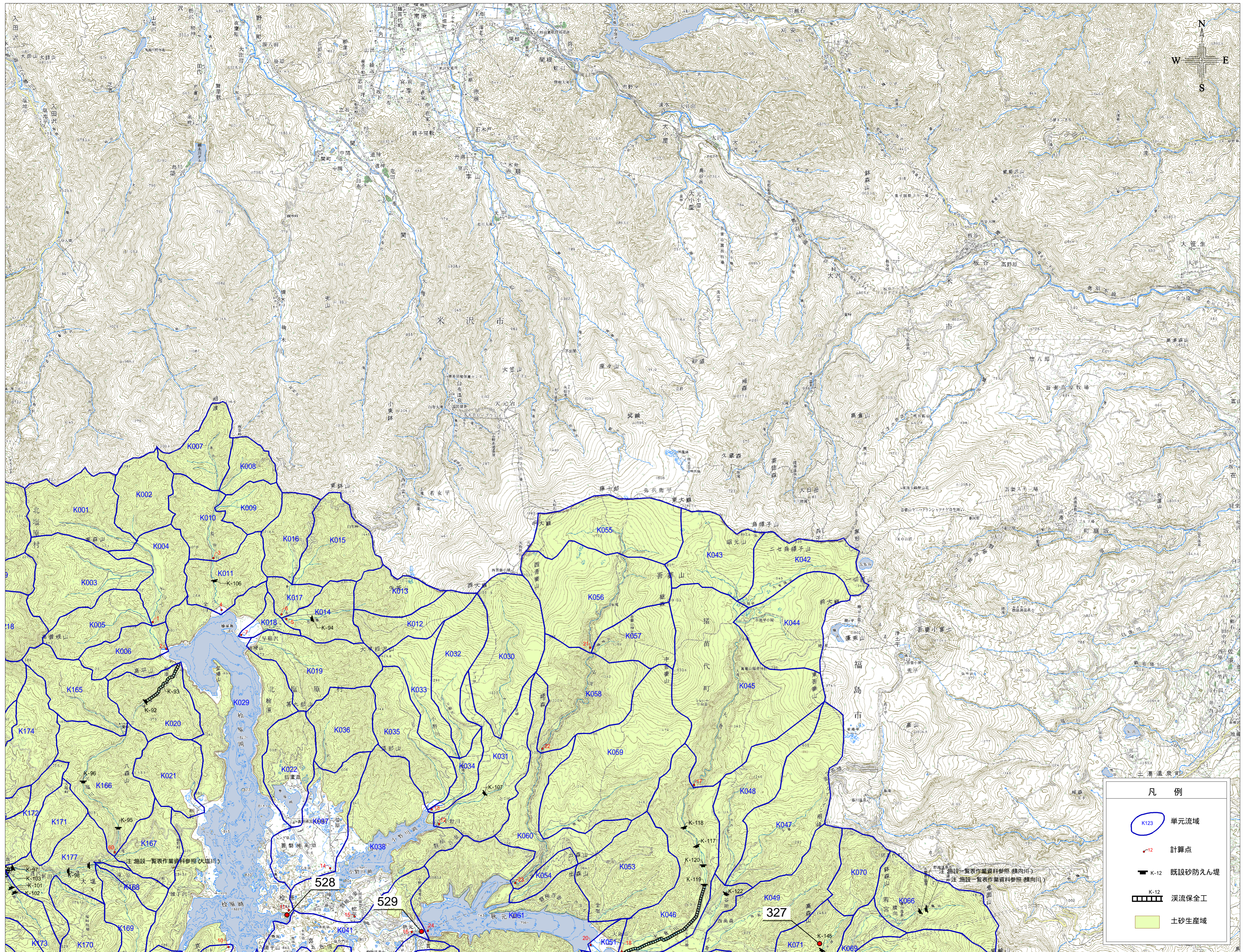
福島県喜多方建設事務所 流域分割及び施設位置図-3/6
