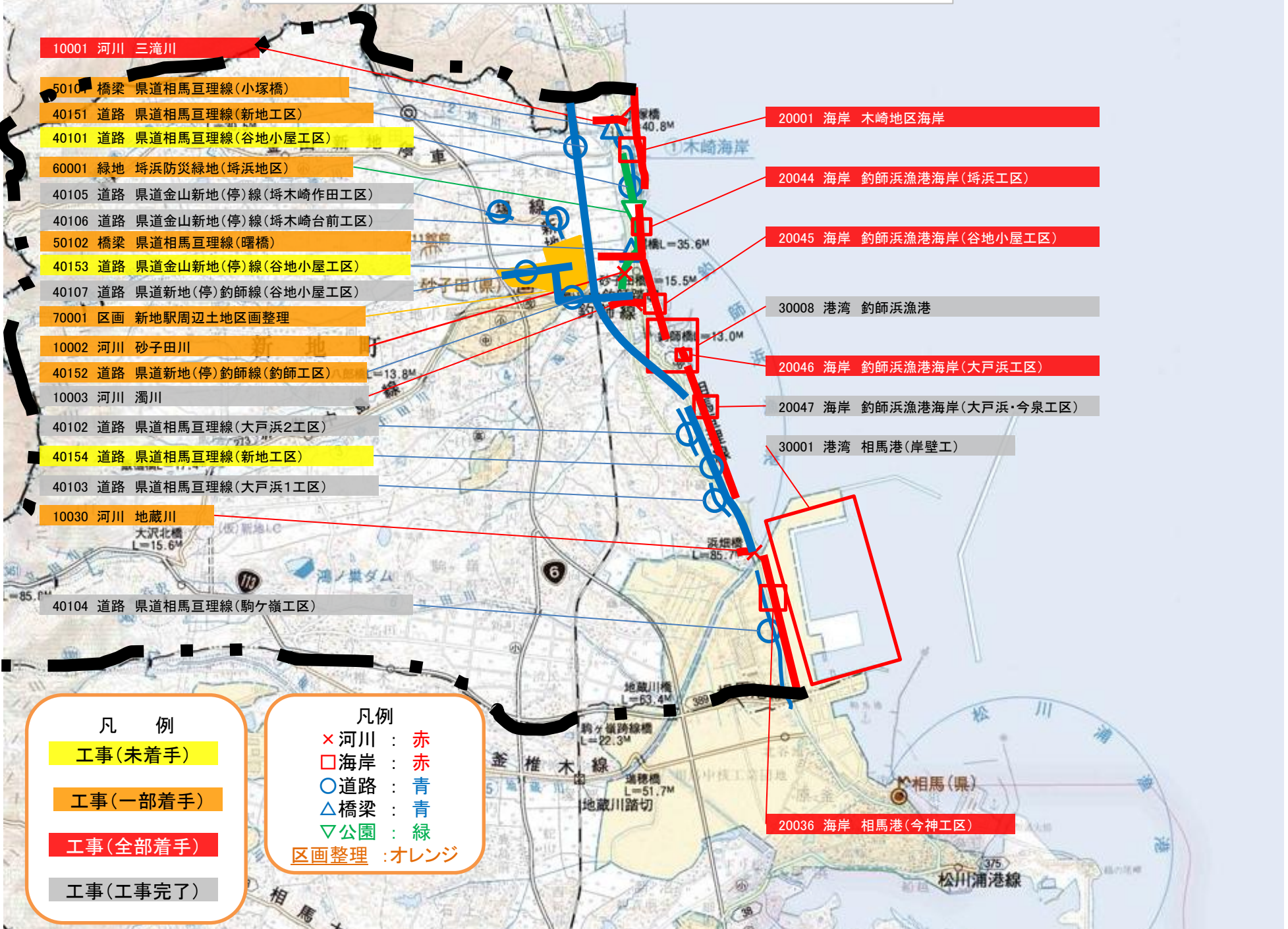
「20044 海岸 釣師浜漁港海岸(埴浜工区)」の施工状況
