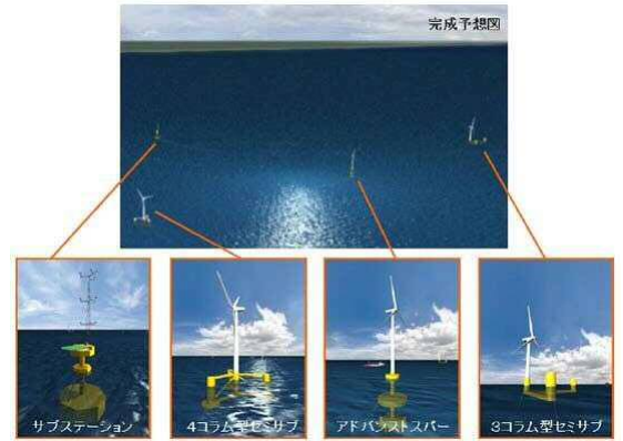
福島県沖における浮体式洋上ウィンドファーム実証研究事業の完成予定図 (丸紅(株)提供)
