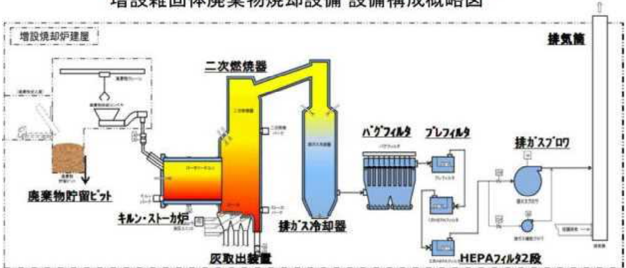
図16 増設雑固体廃棄物焼却設備
