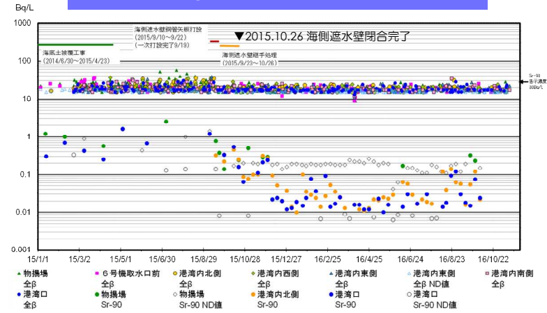
全β、Sr-90濃度推移
