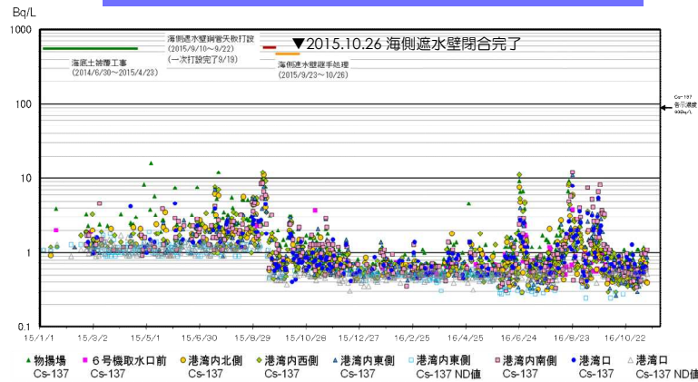
Cs-137濃度推移
