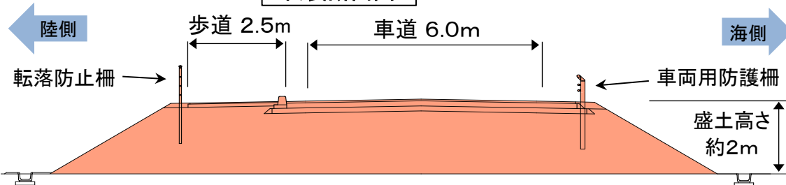
代表断面図
