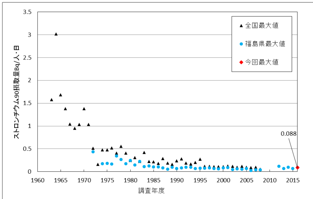
図2 全国及び福島県におけるストロンチウム90摂取量の年度毎の最大値の推移
