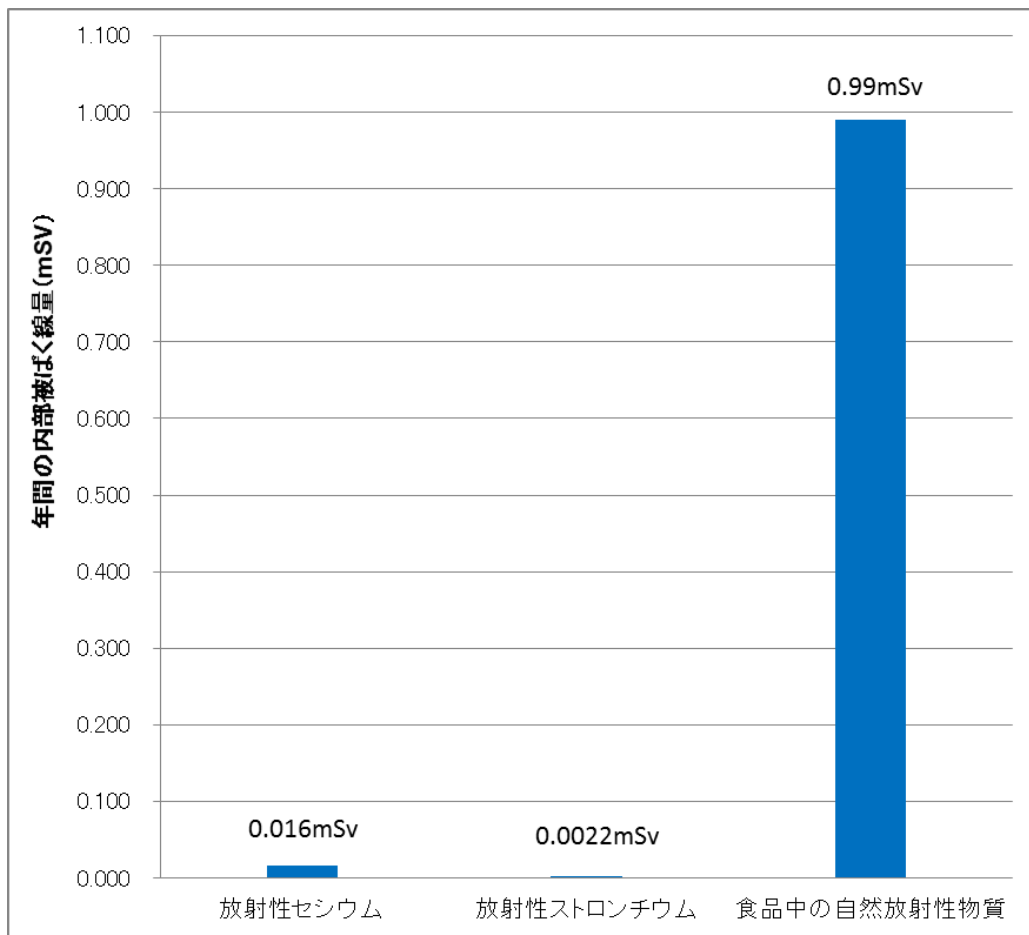
図3 今回調査の最大値と自然放射性物質から受ける内部被ばく線量の比較
