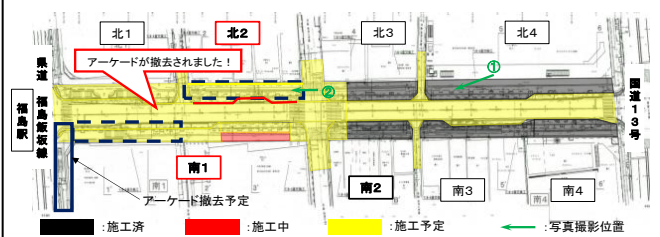
施工箇所図
