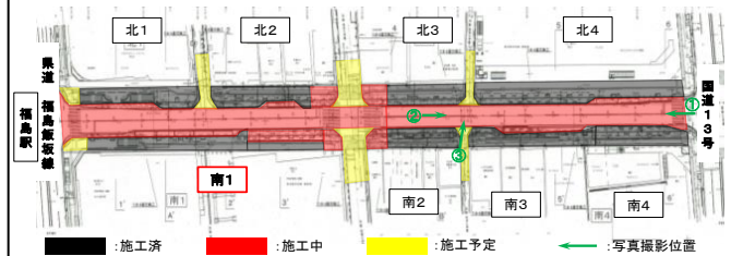
施工箇所図
