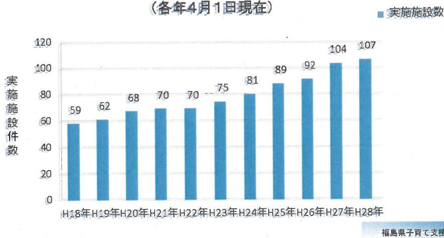
福島県内の地域子育て支援拠点事業実施の推移 (各年4月1日現在)
