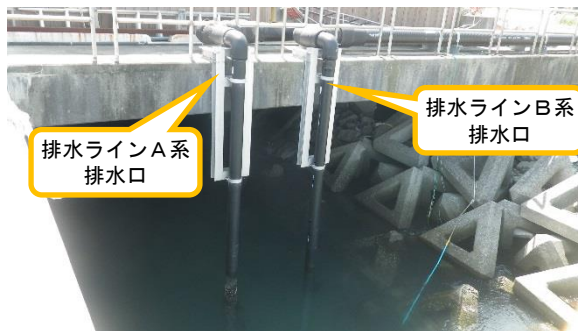
(写真 4 - 2) サブドレン処理水排水口の状況
