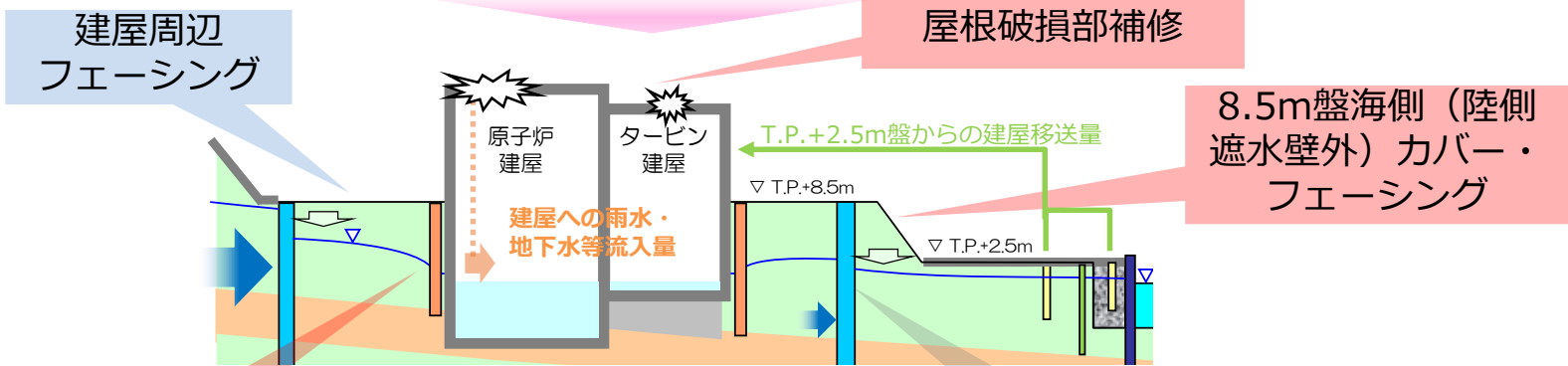
屋根雨水流入対策, T.P.+8.5m盤フェーシング, 建屋滞留水水位・サブドレン水位の低下等
