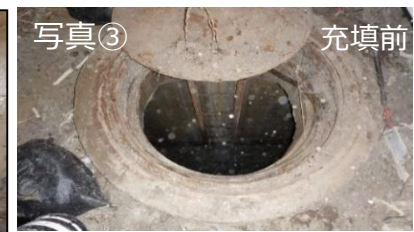
1号機共通配管トレンチ貫通箇所 止水状況
