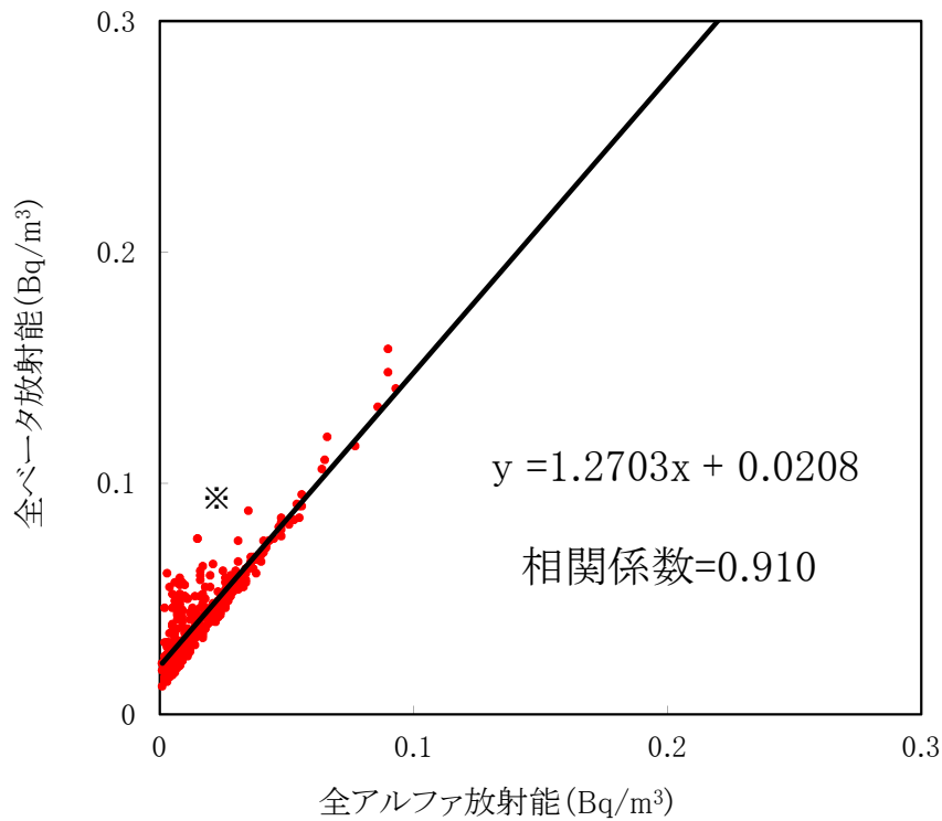
大気浮遊じんの全アルファ・全ベータ放射能の相関図 (MP-3) (平成30年10月～12月)
