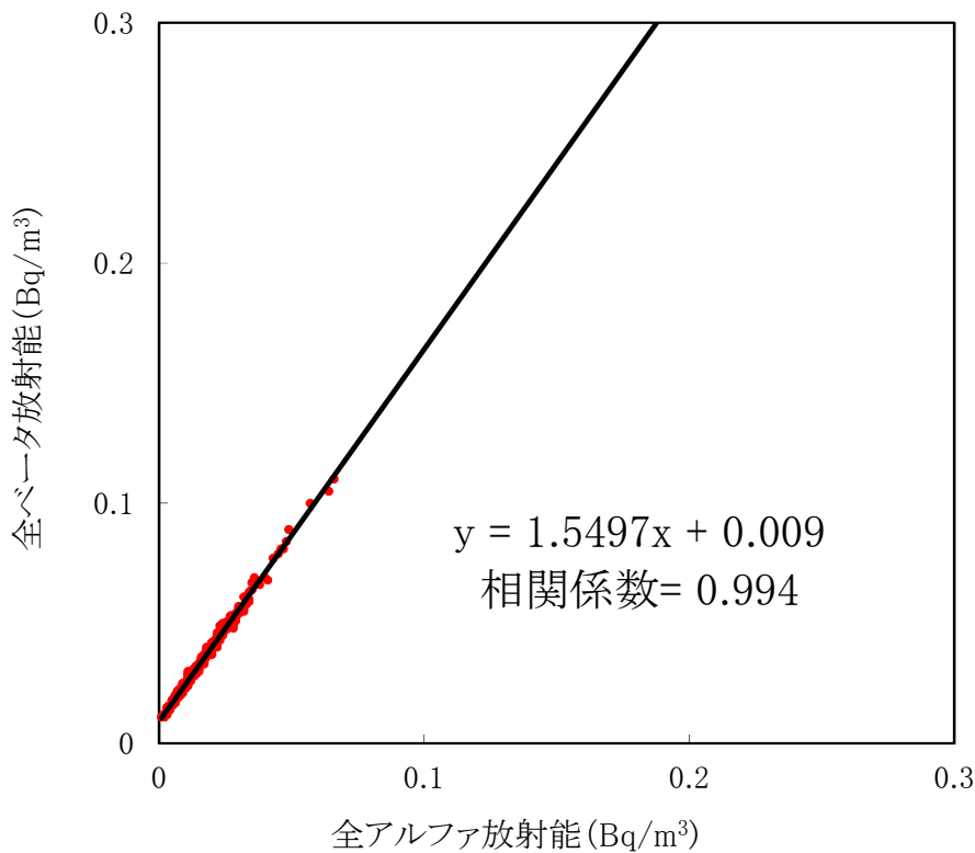
大気浮遊じんの全アルファ・全ベータ放射能の相関図 (MP-7) (平成30年10月～12月)
