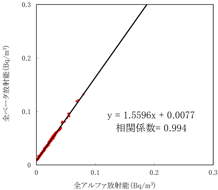
大気浮遊じんの全アルファ・全ベータ放射能の相関図 (MP-1) (平成30年10月～12月)
