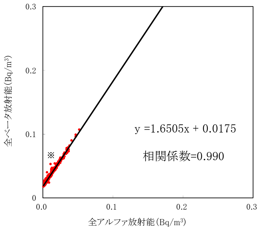
大気浮遊じんの全アルファ・全ベータ放射能の相関図 (MP-8) (平成30年10月～12月)
