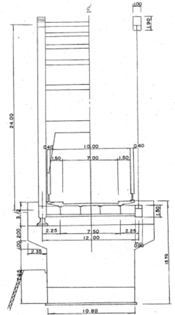
断面図
