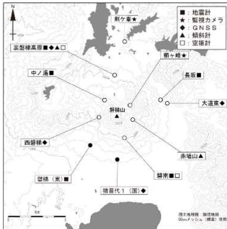
図 1-1 磐梯山観測点配置図（気象庁火山活動解説資料（H30.9）より）
