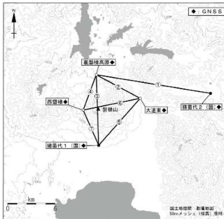
図 1-2 磐梯山 GNSS 観測点配置図（気象庁火山活動解説資料（H30.9）より）
