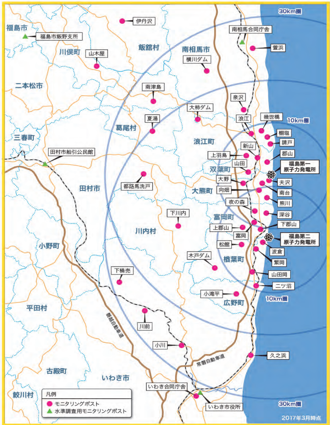
モニタリングポストの配置
