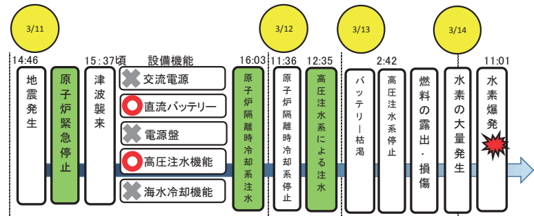
3号機の事故経過
