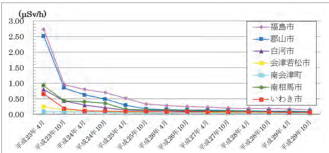
空間線量率の推移
