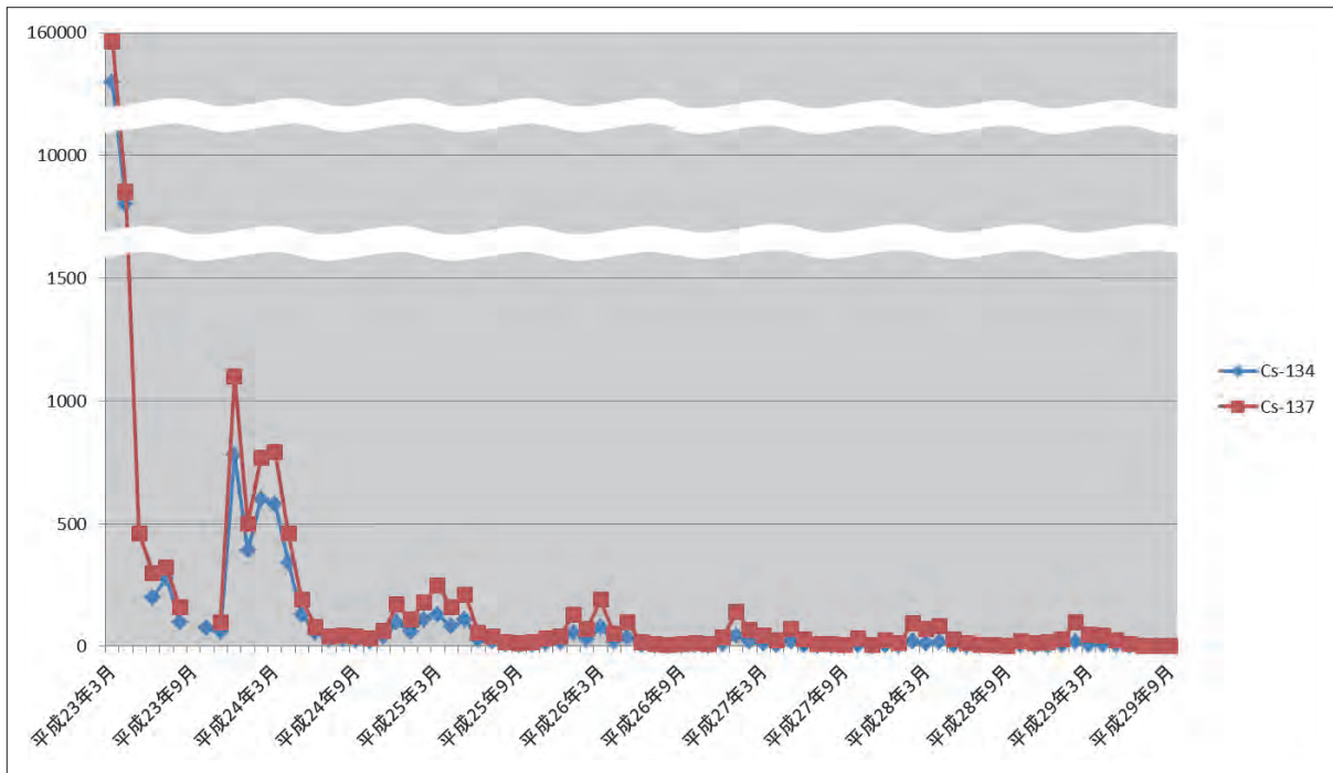
月間降下物中の放射性セシウム濃度の推移（単位 MBq/km 2 = Bq/m 2 ）
