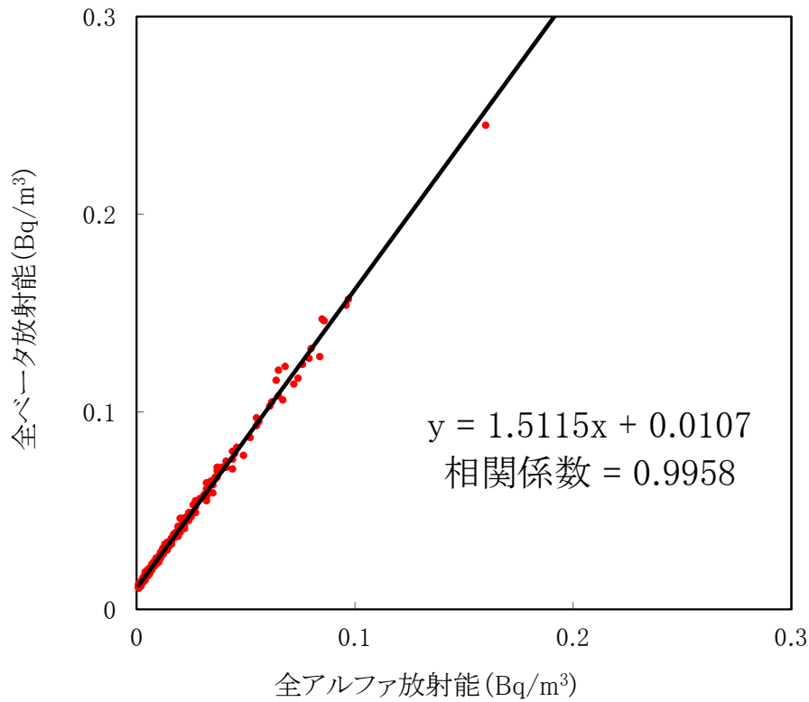
大気浮遊じんの全アルファ・全ベータ放射能の相関図 (MP-1) (平成31年4月～令和元年6月)
