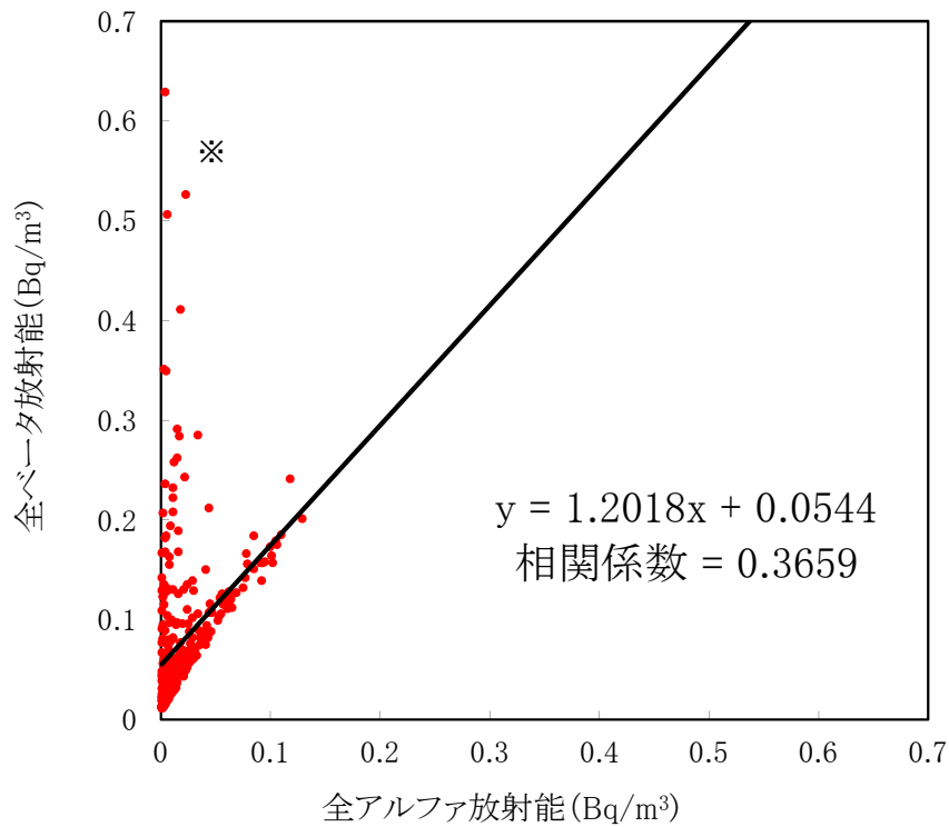
大気浮遊じんの全アルファ・全ベータ放射能の相関図 (MP-3) (平成31年4月～令和元年6月)
