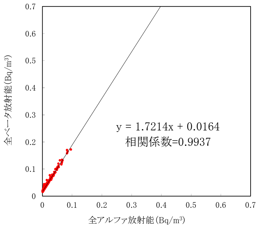
大気浮遊じんの全アルファ・全ベータ放射能の相関図 (MP-8) (平成31年4月～令和元年6月)
