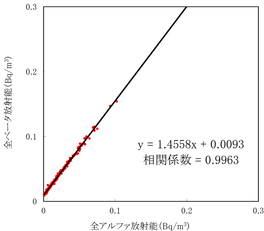
大気浮遊じんの全アルファ・全ベータ放射能の相関図 (MP-7) (平成31年4月～令和元年6月)
