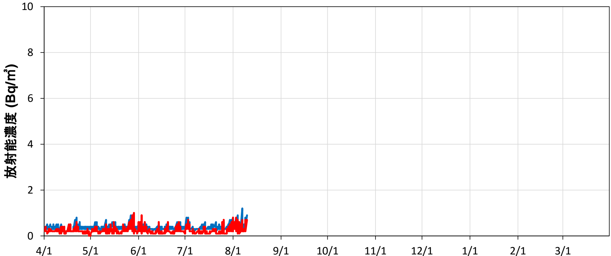
中間貯蔵施設区域境界における大気中のβ線の放射能濃度(連続測定) (2019年4月1日～8月9日)
