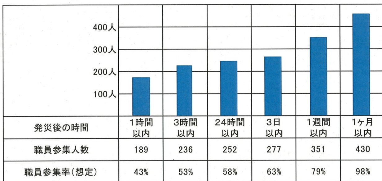
図4 予測結果
