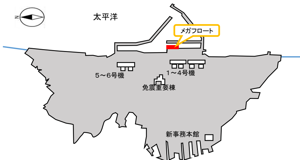
図1 福島第一原子力発電所構内概略図
