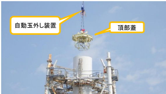
(写真 1 - 3) 頂部蓋設置中の状況②
