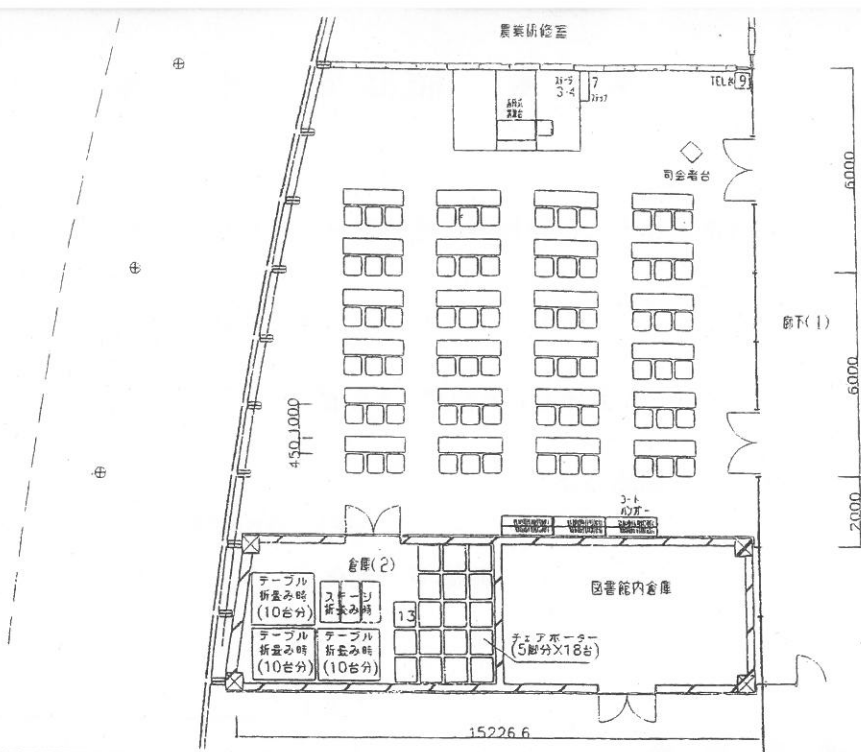
大会議室 基本レイアウト SCALE 1:100 DATE 福島県農業総合研究センター JOB No. DRAWN BY DESIGNED BY レイアウト平面図 DRAWING No. CHECKED BY DATE 3311
