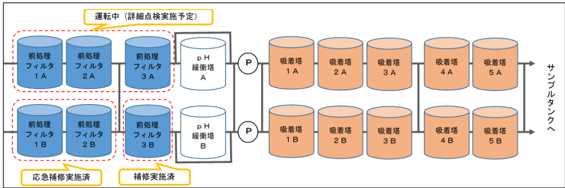
(図2) サブドレン他浄化設備概略図
