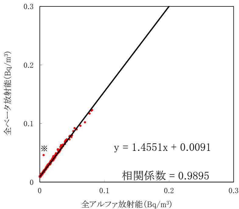
大気浮遊じんの全アルファ・全ベータ放射能の相関図 (MP-7) (令和2年4月～6月)
