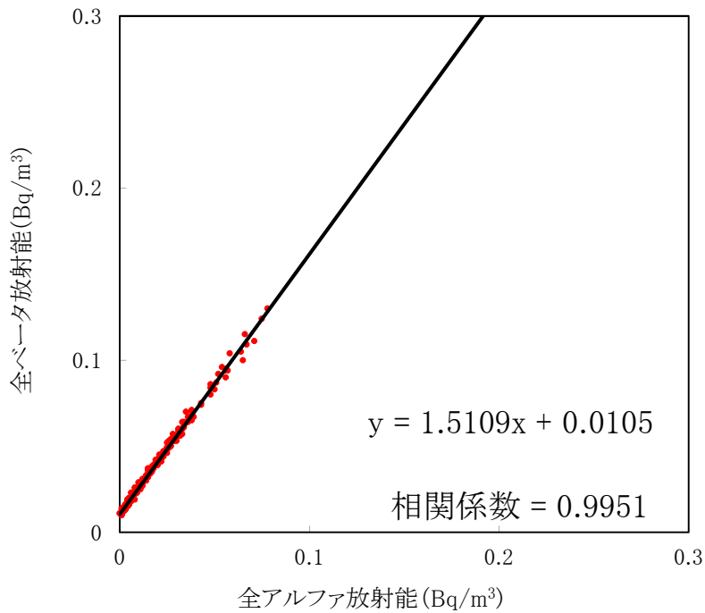
大気浮遊じんの全アルファ・全ベータ放射能の相関図 (MP-1) (令和2年4月～6月)
