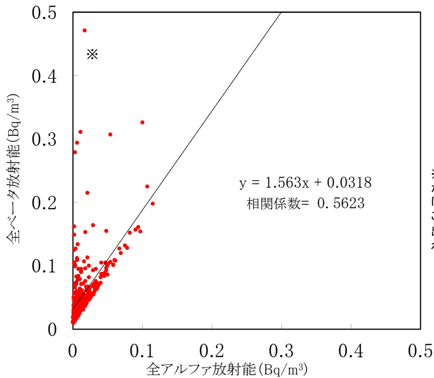
大気浮遊じんの全アルファ・全ベータ放射能の相関図 (MP-3) (令和2年4月～令和2年6月)
