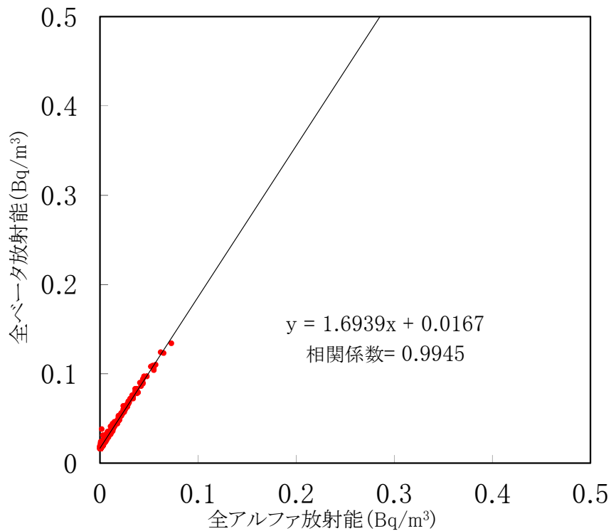
大気浮遊じんの全アルファ・全ベータ放射能の相関図 (MP-8) (令和2年4月～令和2年6月)
