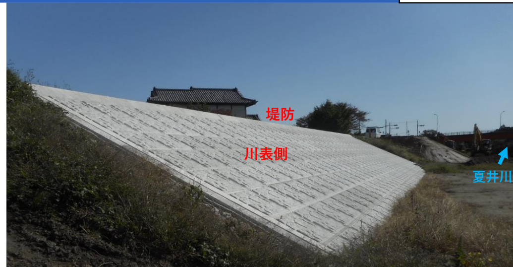
川表側 コンクリート張ブロック完了 (5月末)
