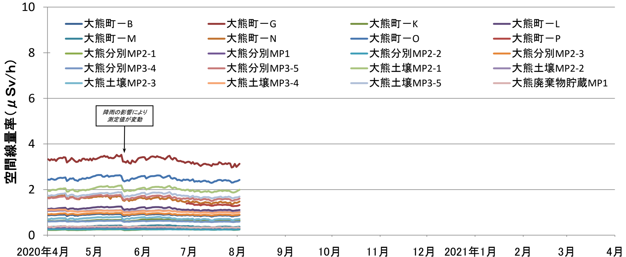
空間線量率の推移（連続測定）（2020年4月1日～8月2日）
