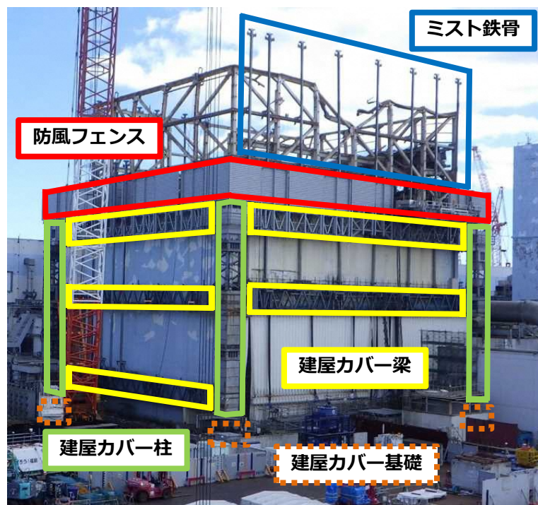
1号機原子炉建屋全景 (2020年3月時点)
