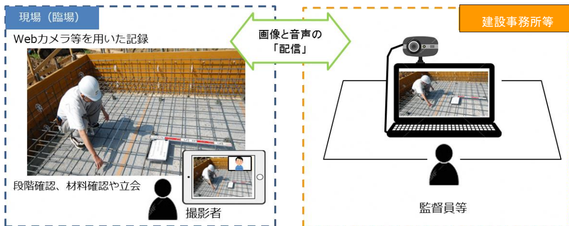
図 2-1 機器構成(例)
