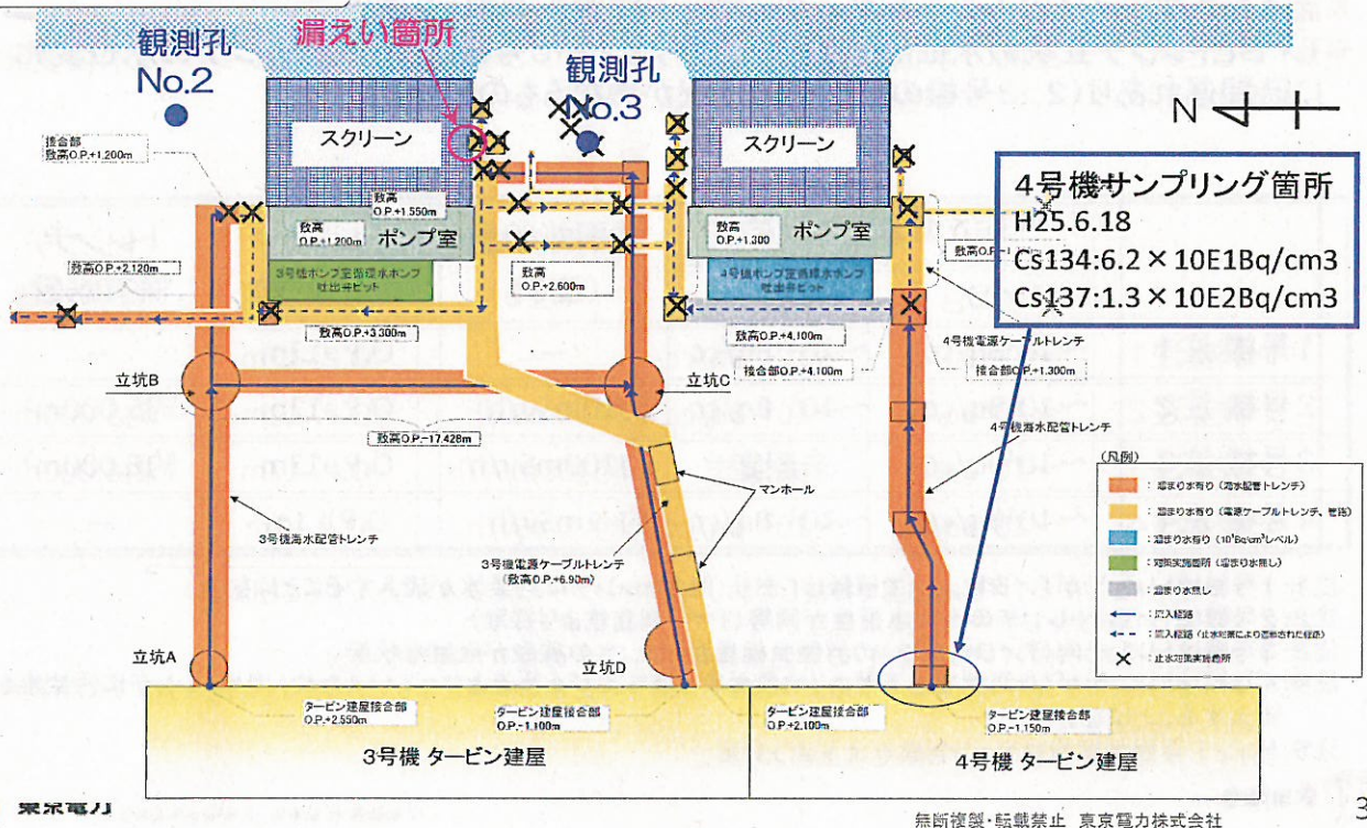
3/4号機平面図
