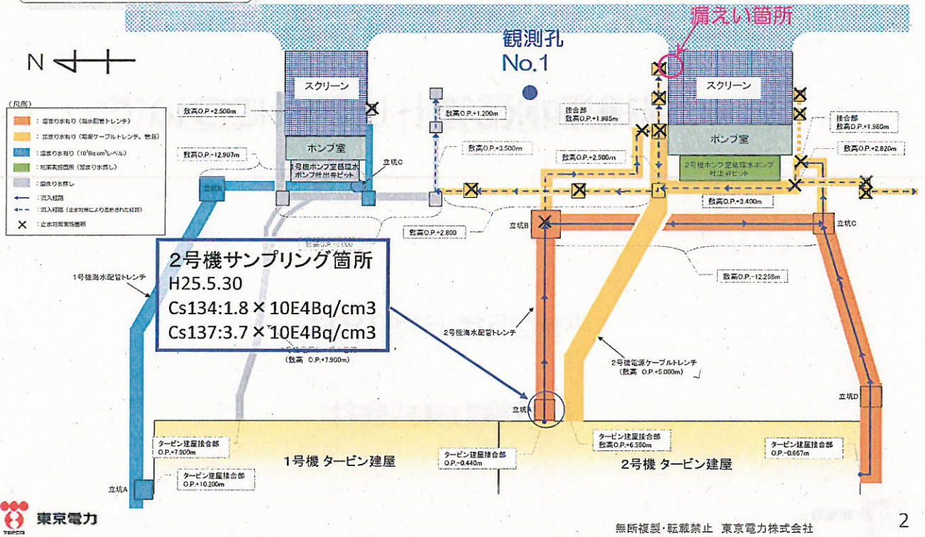
1/2号機平面図
