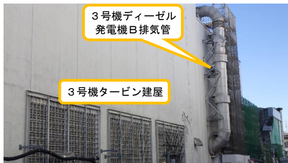
(写真2-2) 3号機ディーゼル発電機排気管（3号 機タービン建屋北側）の状況 (北東側から撮影)
