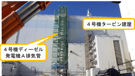
(写真1) 4号機ディーゼル発電機排気管の 除却工事用足場の設置状況 (東側から撮影)
