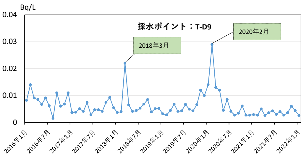
原子力規制委員会調査 沿岸海域海水Cs-137濃度推移
