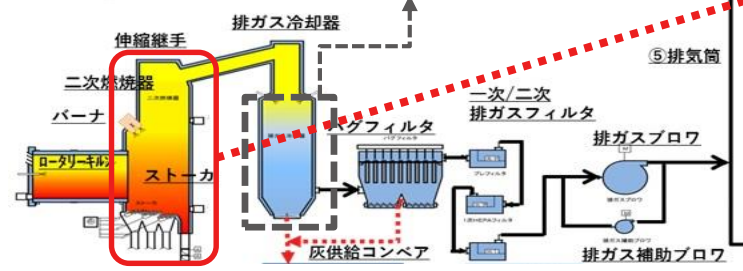
増設雑固体廃棄物焼却設備系統図
