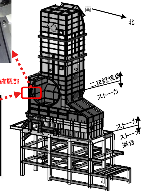
二次燃焼器・ストーカ立体図
