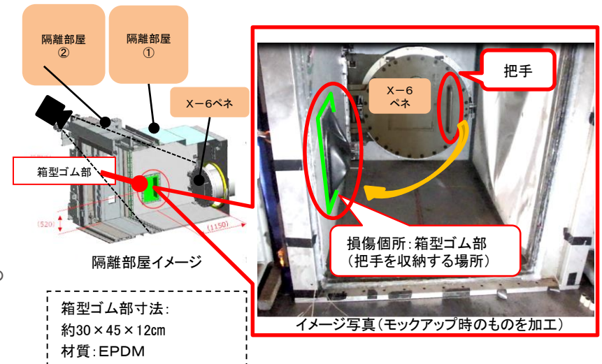
隔離部屋の対策(箱型ゴム部損傷)
