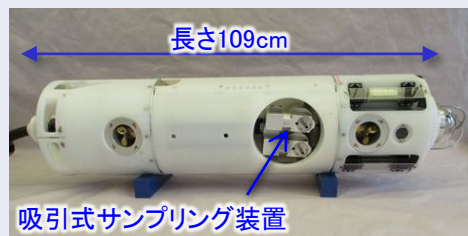
調査装置ROV-E(堆積物サンプリング用)
