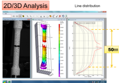
<観察例1> 丸棒引張試験
