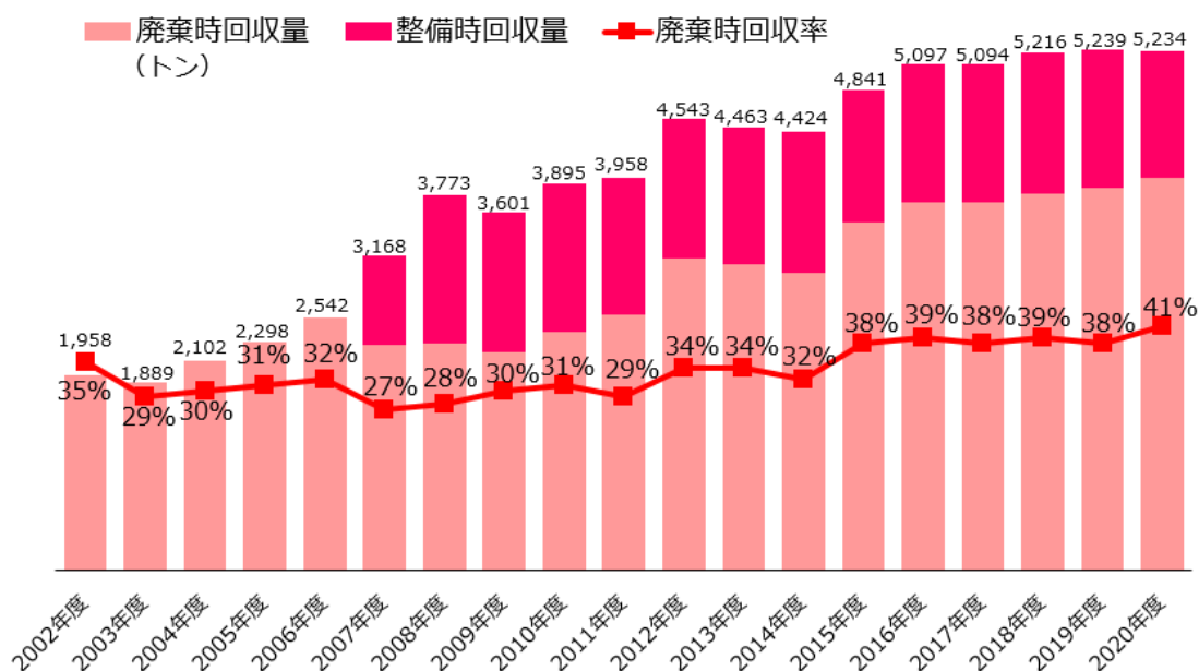
図33 全国の業務用冷凍空調機器からのフロン類回収量等 (2020年度)
