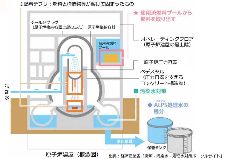
原子炉建屋（概念図） 出典：経済産業省「廃炉・汚染水・処理水対策ポータルサイト」
