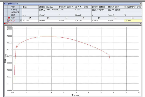
引張試験の結果
