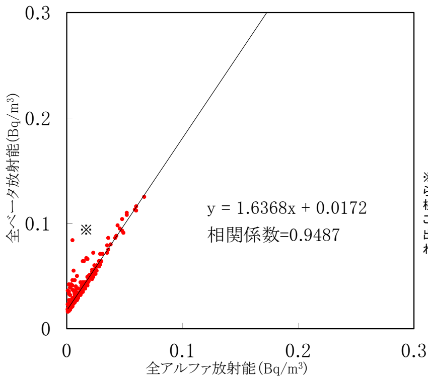
大気浮遊じんの全アルファ・全ベータ放射能の相関図 (MP-8) (令和5年1月～令和5年3月)
