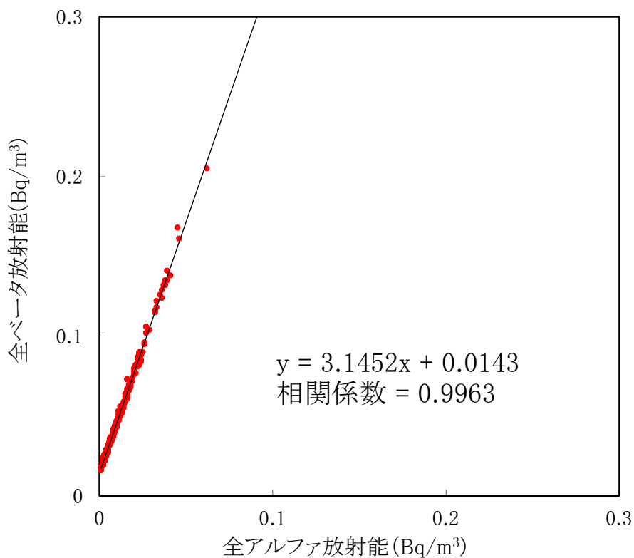
大気浮遊じんの全アルファ・全ベータ放射能の相関図 (MP-7) (令和5年1月～令和5年3月)
