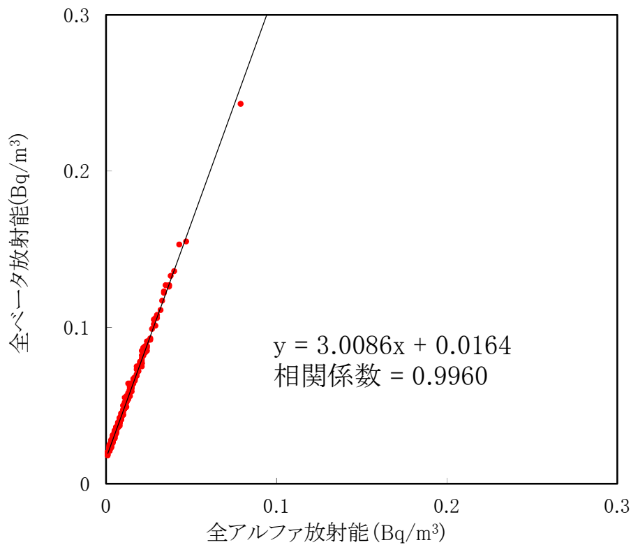
大気浮遊じんの全アルファ・全ベータ放射能の相関図 (MP-1) (令和5年1月～令和5年3月)
