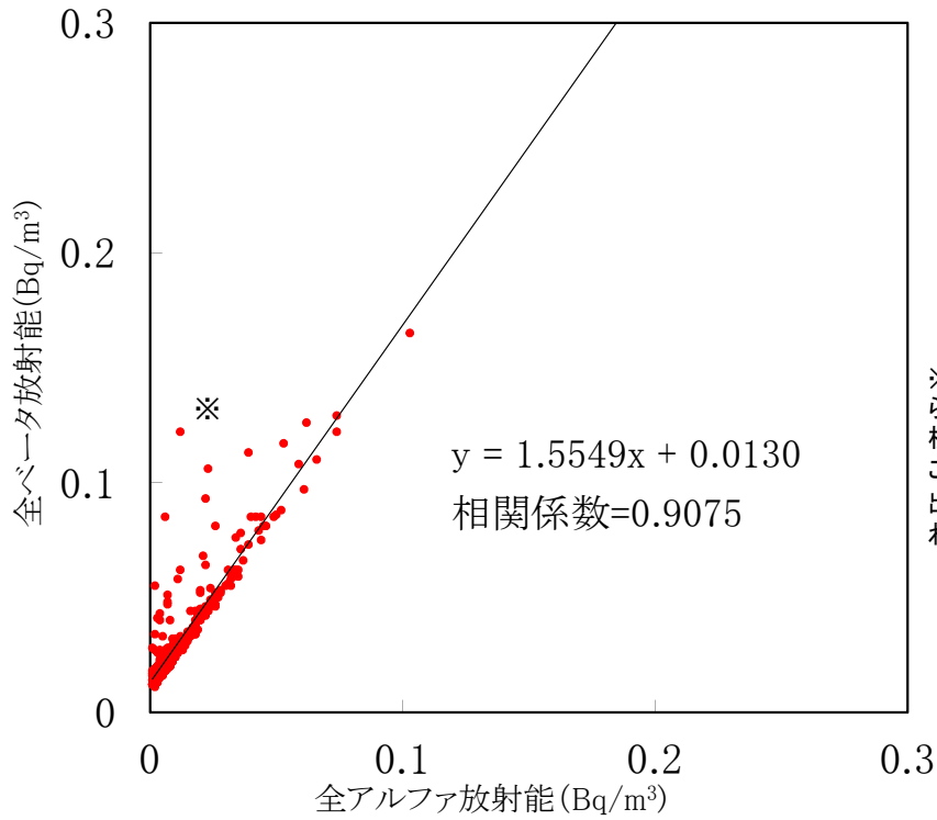
大気浮遊じんの全アルファ・全ベータ放射能の相関図 (MP-3) (令和5年1月～令和5年3月)
