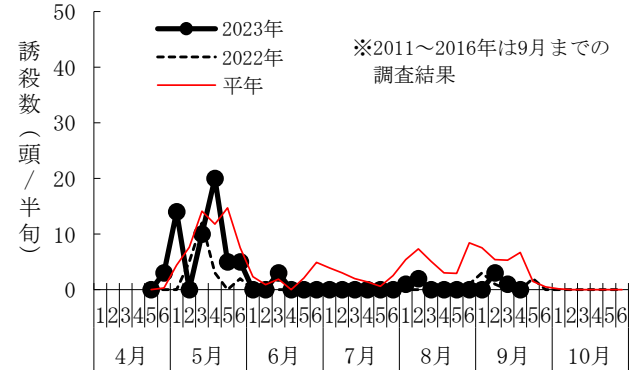
図6 スモモヒメシクイの誘殺状況(会津美里町)
