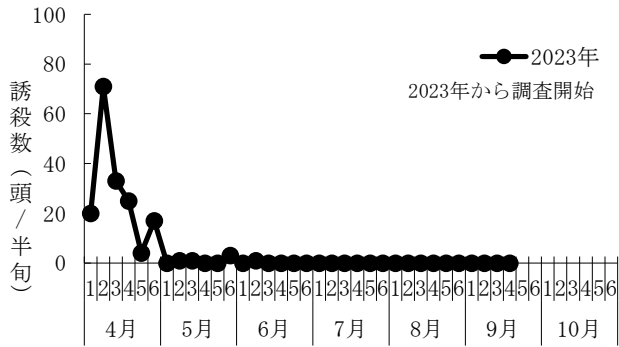
図1 モモハマグリガの誘殺状況(伊達市)
