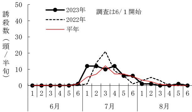
図11 ヒメボクトウの誘殺状況(須賀川市)
