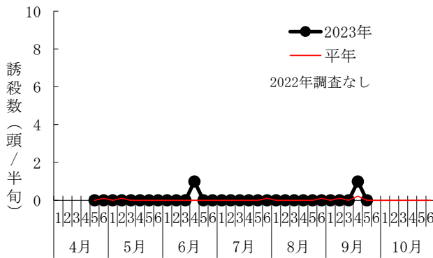
図5 スモモヒメシクイの誘殺状況(伊達市)
