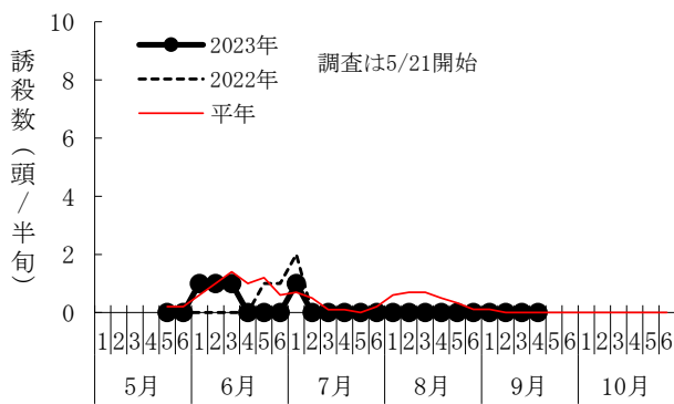
図7 モモシクイガの誘殺状況(会津若松市)
