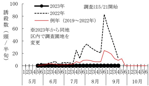
図10 コスカシバの誘殺状況(福島市)
