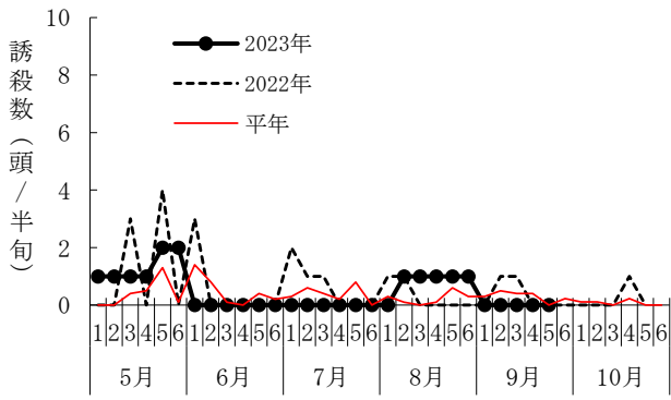
図9 リンゴカクモンハマキの誘殺状況(須賀川市)
