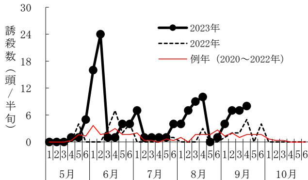
図8 モモゴマダラノメイガの誘殺状況(福島市)
