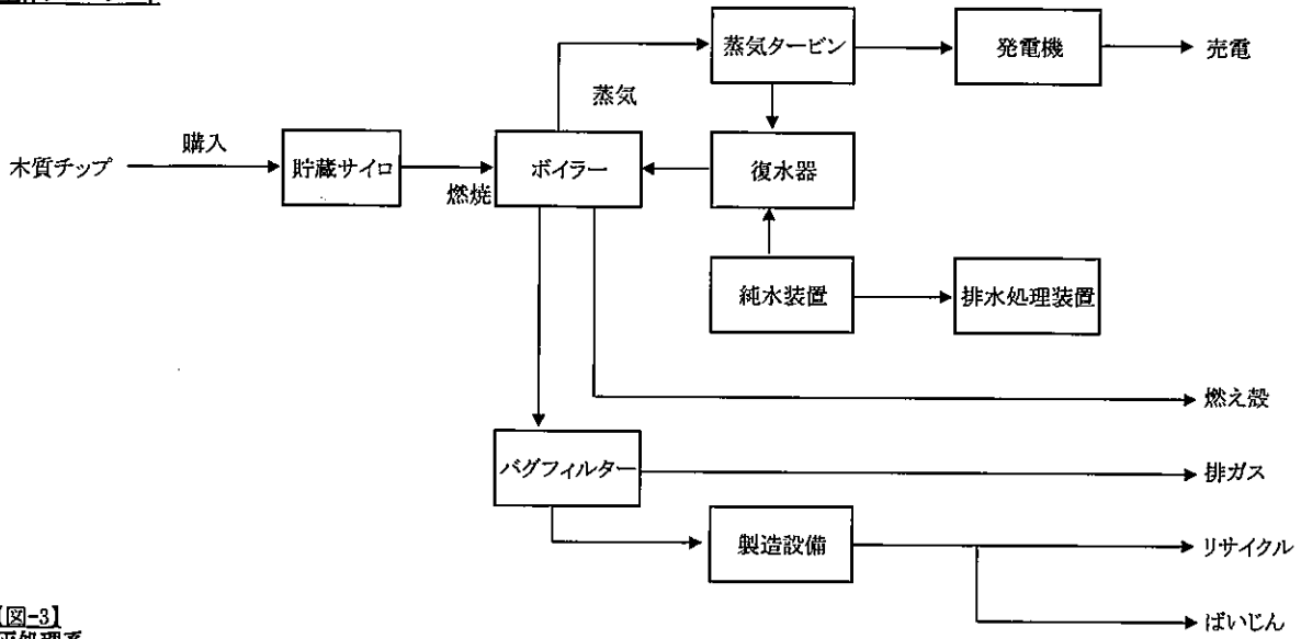
【図-2】 全体フローシート
