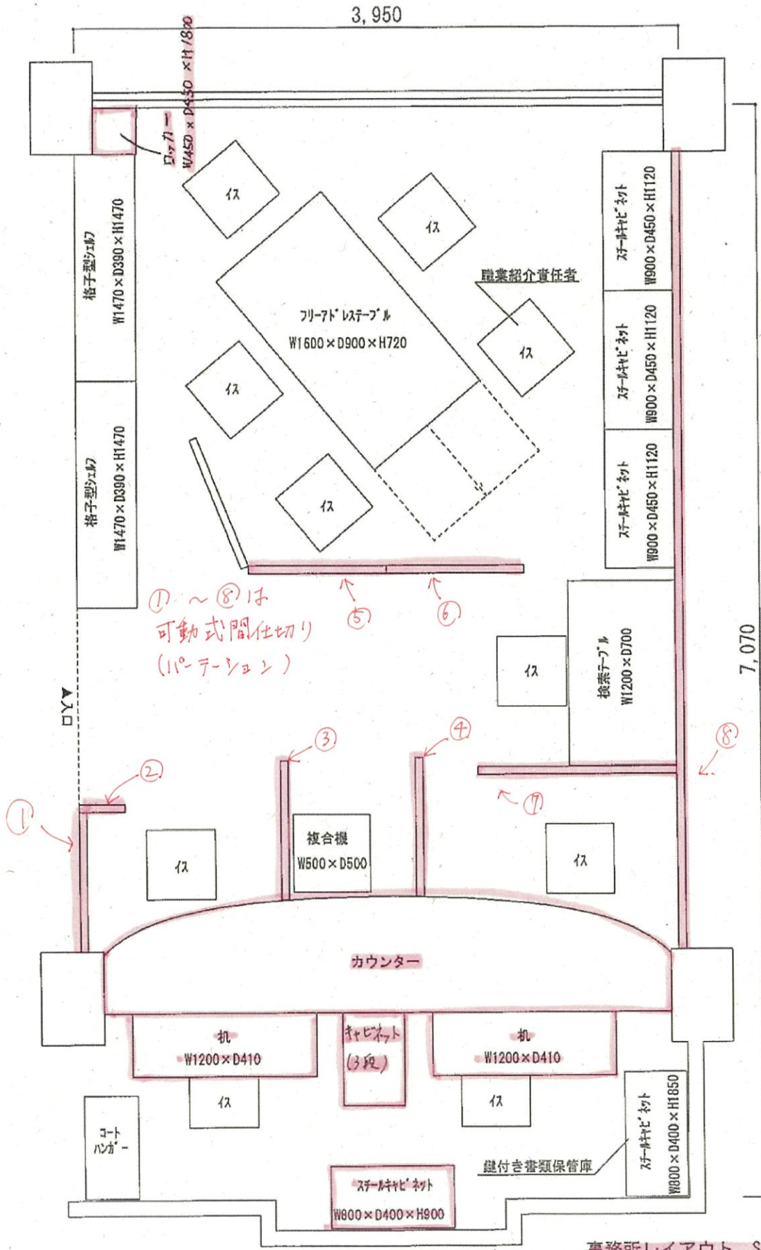
事務所レイアウト S=1/30 床面積：27.92㎡
