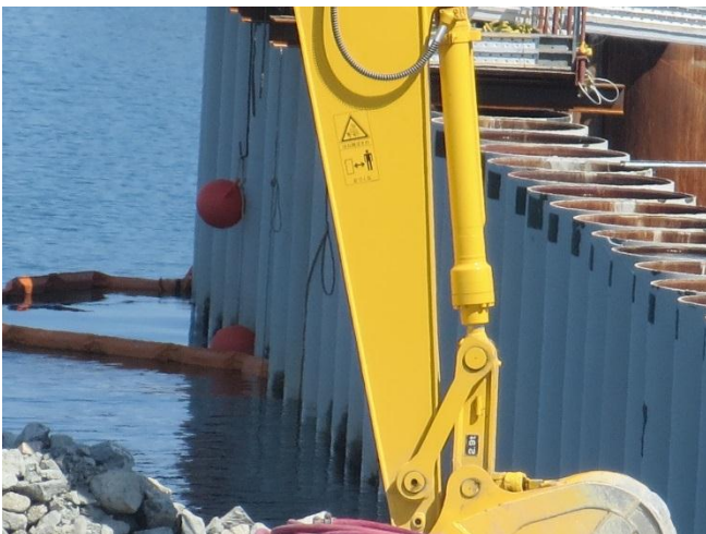
海側遮水壁
